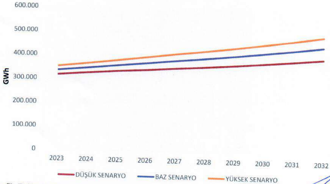
Grafik: Türkiye Elektrik Talep Tahmini Kaynak: TEİAŞ
