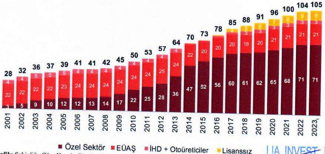
Grafik: Sahipliğe Göre Kurulu Güç Payları Kaynak: PWC, TEİAŞ
